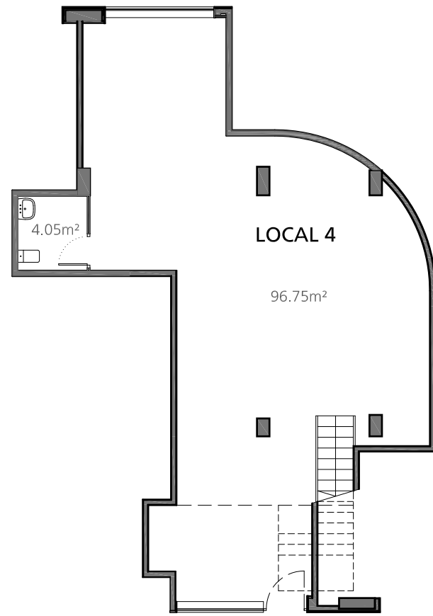
PLANTA BAIXA
